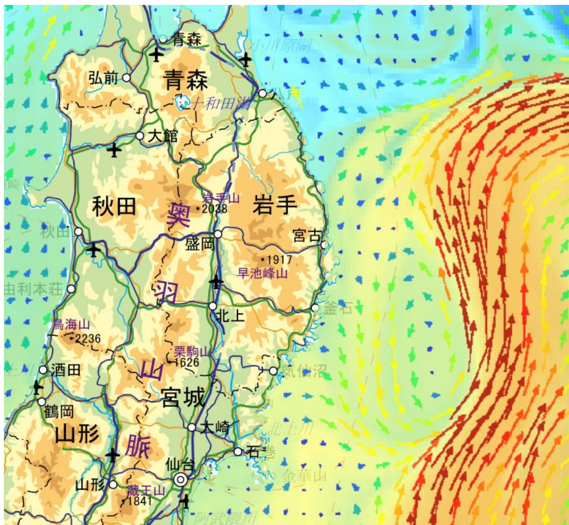
令和6年5月7日13時00分の潮流図(表面の解析値) 提供:宇宙航空研究開発機構・海洋研究開発機構(JAXA)
