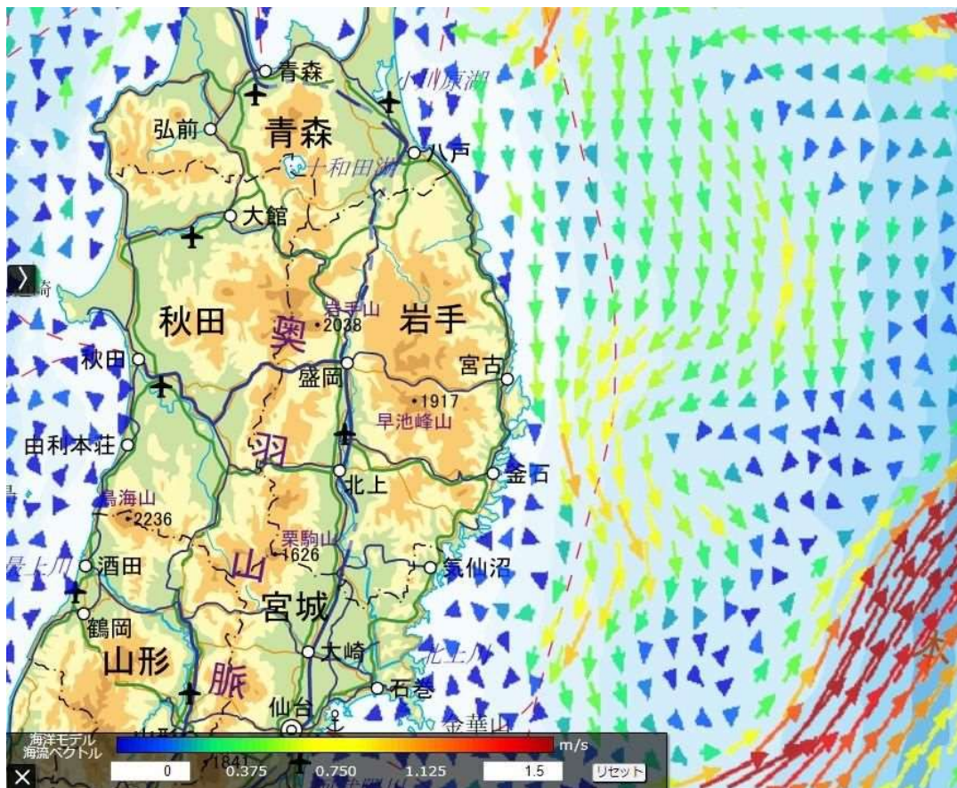
令和6年10月13日12時00分の潮流予想図（表面の解析値） 提供：宇宙航空研究開発機構・海洋研究開発機構（JAXA）
